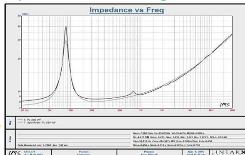
Impedance/Phase
