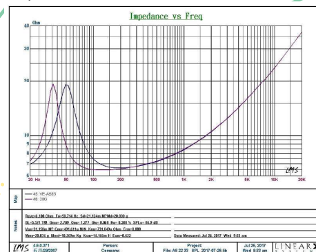
Impedance/Phase
