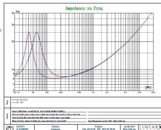
Impedance/Phase
