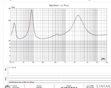
Impedance/Phase
