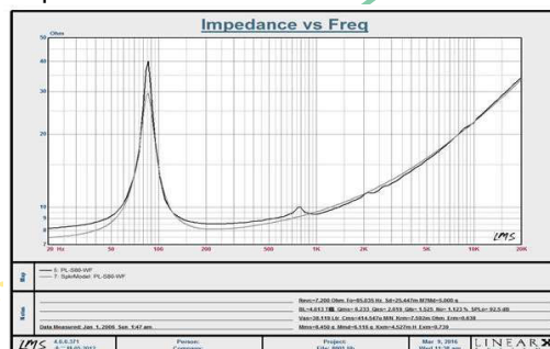
Impedance/Phase
