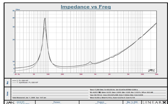
Impedance/Phase
