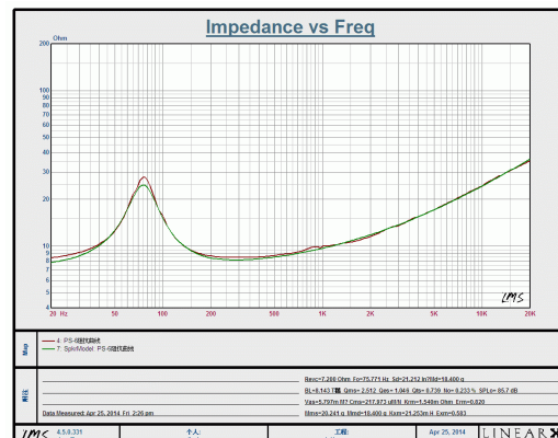
Impedance/Phase
