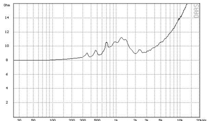
Impedance/Phase
