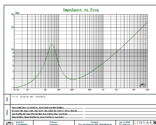
Impedance/Phase
