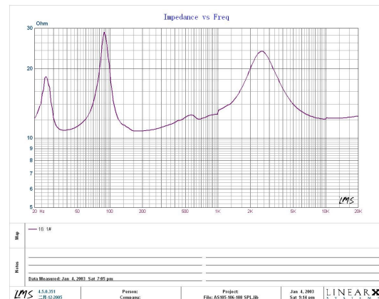
Impedance/Phase
