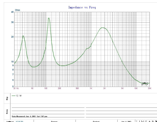
Impedance/Phase
